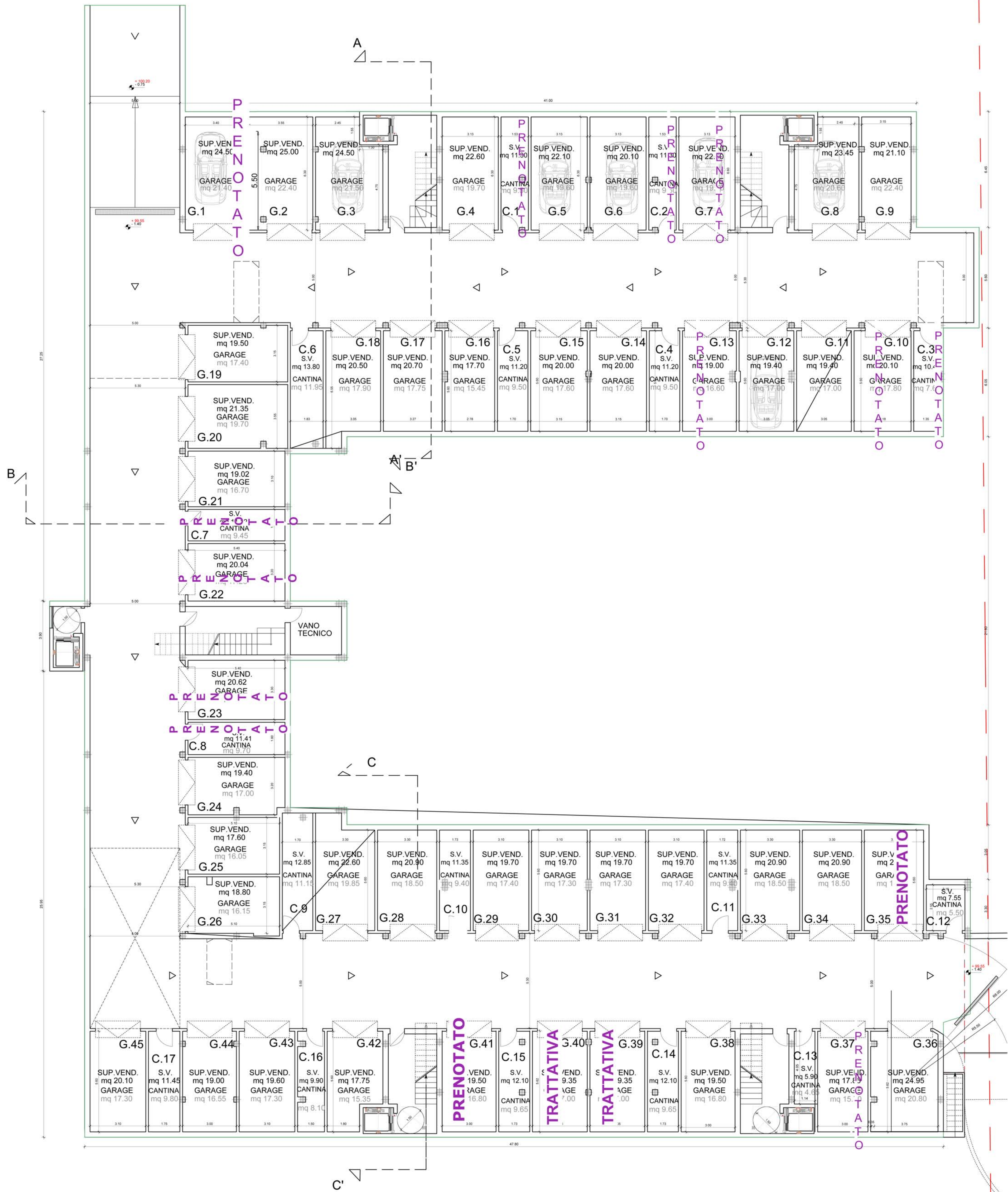
Pianta piano Interrato
