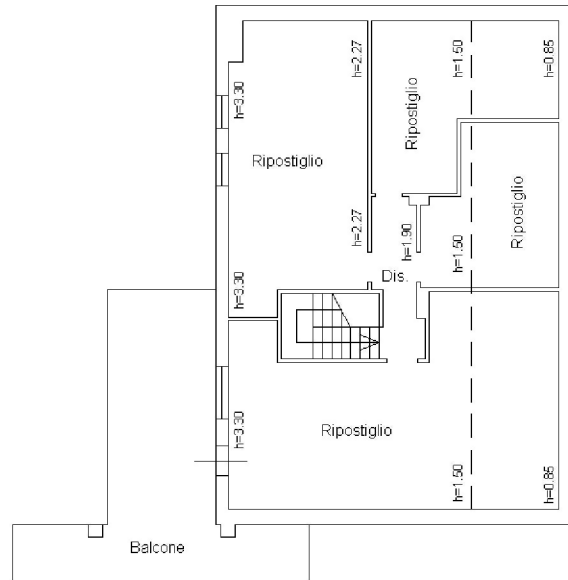
PIANO QUARTO (Sottotetto)
